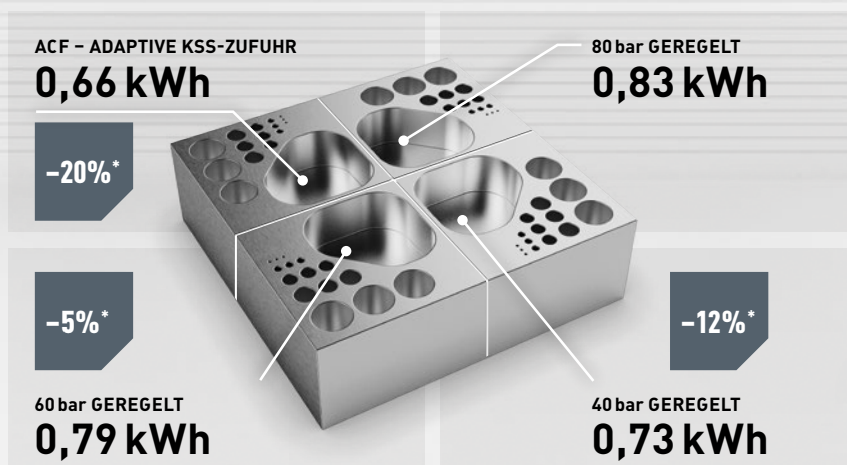
Energiewerte der Gesamtmaschine für die Bearbeitung des gezeigten Bauteils auf der DMU 65 FDS monoBLOCK.
